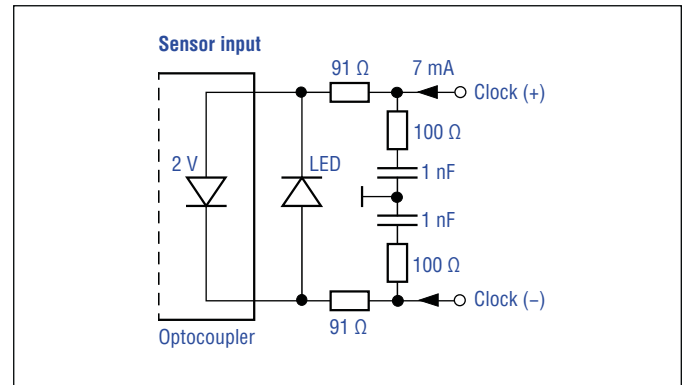
Fig. 26: Input wiring clock (+)/clock (-)
